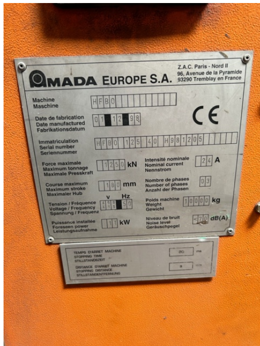
PLAQUE CONSTRUCTEUR
